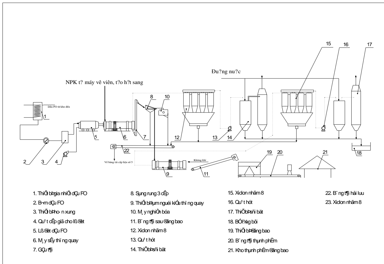
Hình 4. Sơ đồ quy trình công nghệ hệ thống thu hồi, xử lý bụi trong sản xuất NPK
